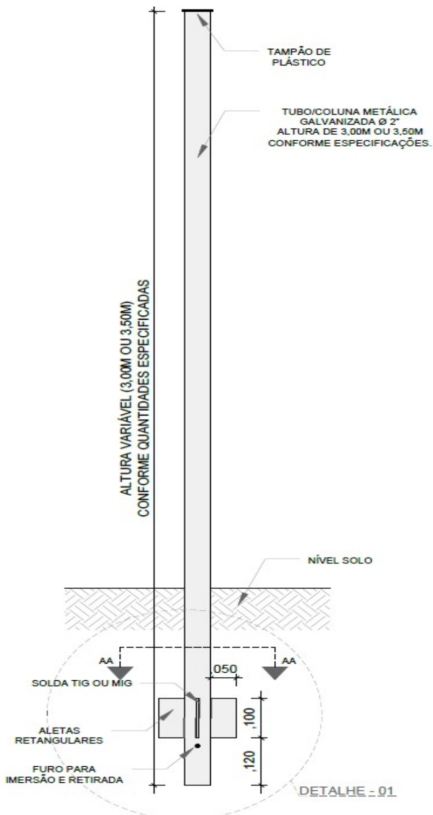
FIGURA 6 – DETALHE FRONTAL DA COLUNA METÁLICA 2". FONTE: DET/SMST/PMBV
