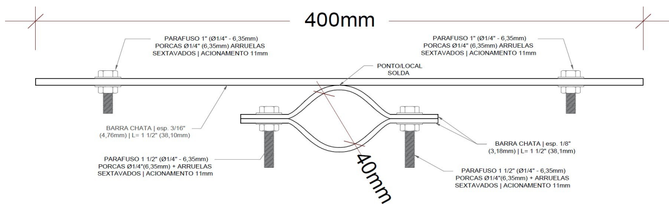
FIGURA 1 – VISTA SUPERIOR DA ABRAÇADEIRA. FONTE: DET/SMST/PMBV
